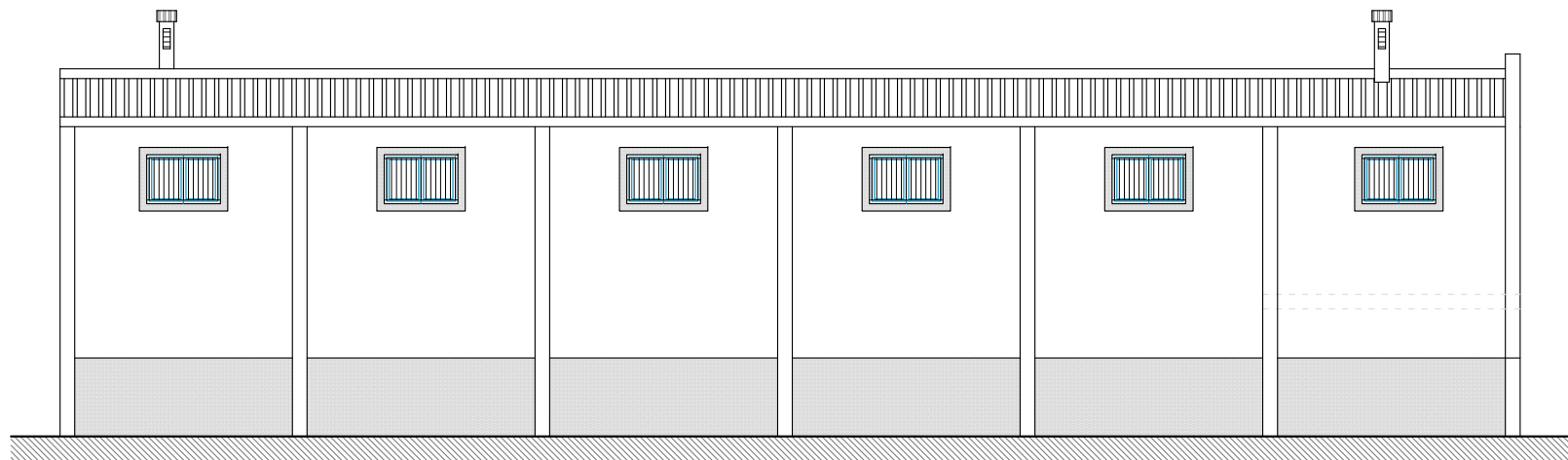
ALZADO SUR
