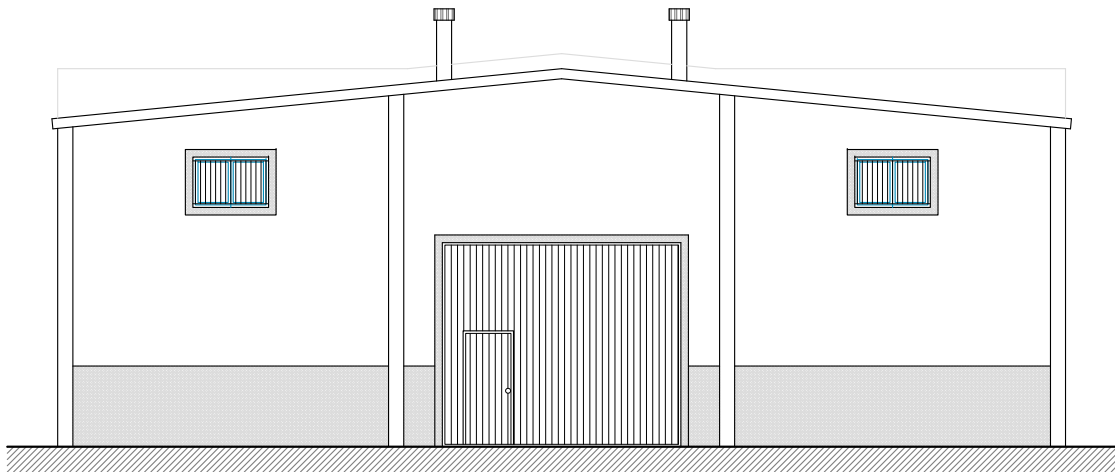
ALZADO OESTE
