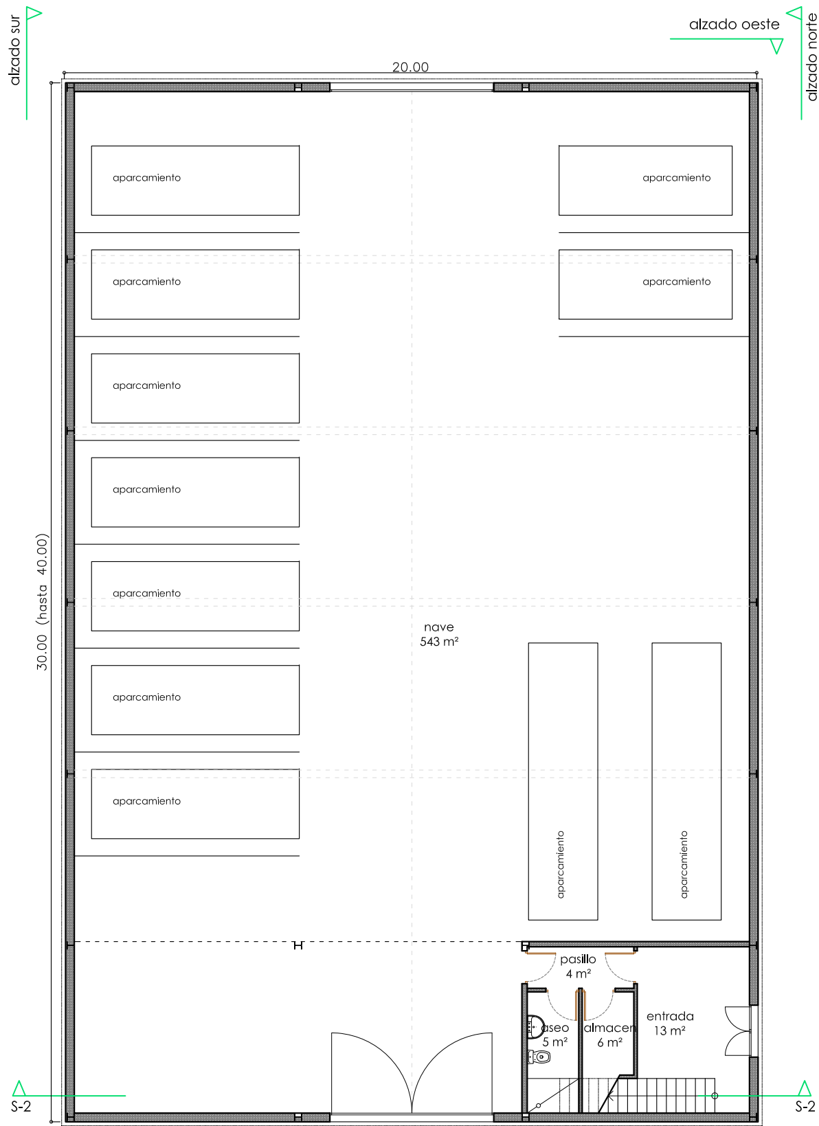
PLANTA BAJA
