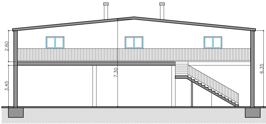
SECCION 1
