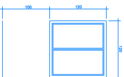
TIPO V2 5 UNIDADES. ALUMINIO IMITACIÓN MADERA ROTURA DE PUENTE TÉRMICO
