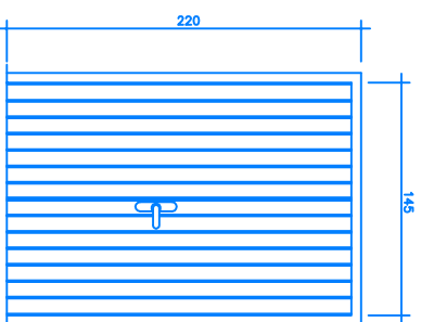
TIPO P4 2 UNIDADES. MADERA PINO TRATADA MANIVELA ACERO INOXIDABLE
