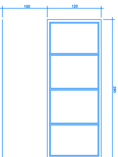
TIPO V3 1 UNIDAD. ALUMINIO IMITACIÓN MADERA ROTURA DE PUENTE TÉRMICO
