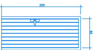
TIPO P2 2 UNIDADES. MADERA PINO TRATADA MANIVELA ACERO INOXIDABLE
