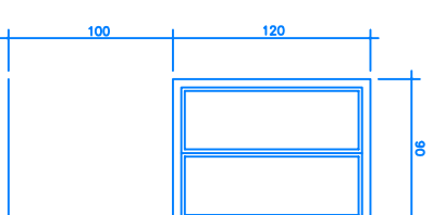
TIPO V5 ↑ UNIDAD. ALUMINIO IMITACION MADERA ROTURA DE PUENTE TÉRMICO
