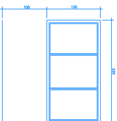
TIPO V4 1 UNIDAD. ALUMINIO IMITACIÓN MADERA ROTURA DE PUENTE TÉRMICO
